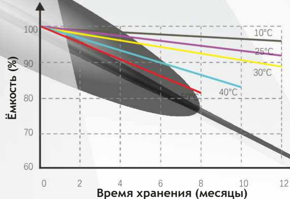
Саморазряд при хранении
