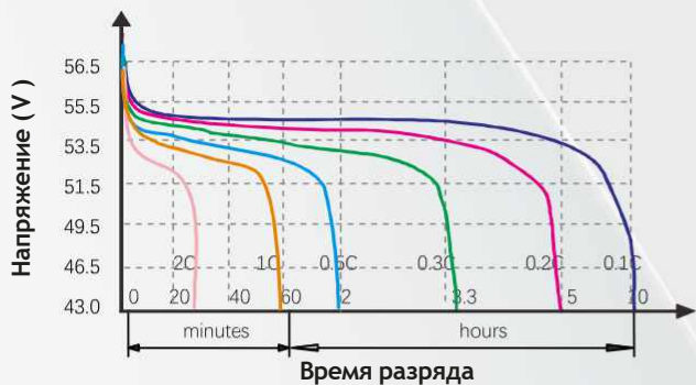
Графики разряда разными токами при 25 °C
