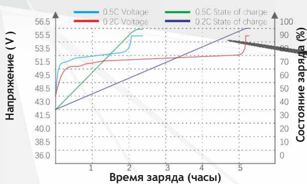
Кривая состояния заряда при 25 °C
